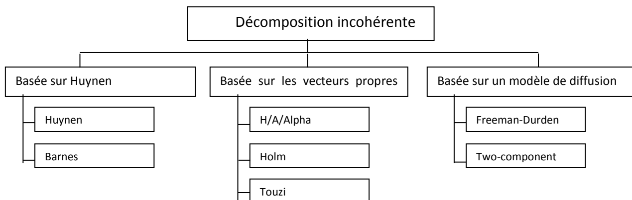
Figure 18 : Décompositions incohérentes
