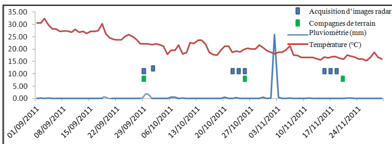
Figure 39. Diagramme récapitulant la pluviométrie enregistré et la date d'acquisition des images et des campagnes de terrain
