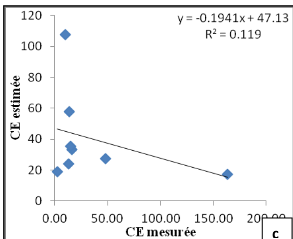
Les courbes de la validation croisée pour les modèles des campagnes 1-2 pour le site tunisien (25°.7) a) HH b) HV et c) VV
