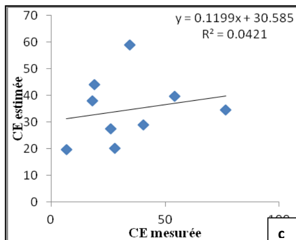
Les courbes de la validation croisée pour les modèles des campagnes 2-3 pour le site tunisien (25°.7) a) HH b) HV et c) VV
